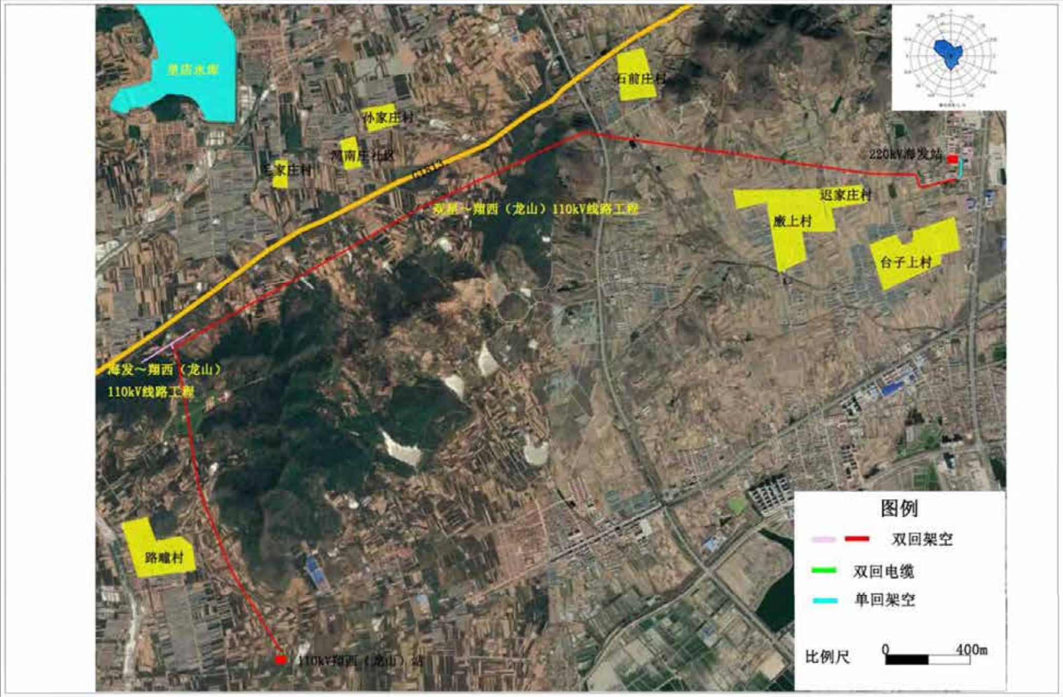
附图5 本工程环评阶段站址及输电线路路径图
