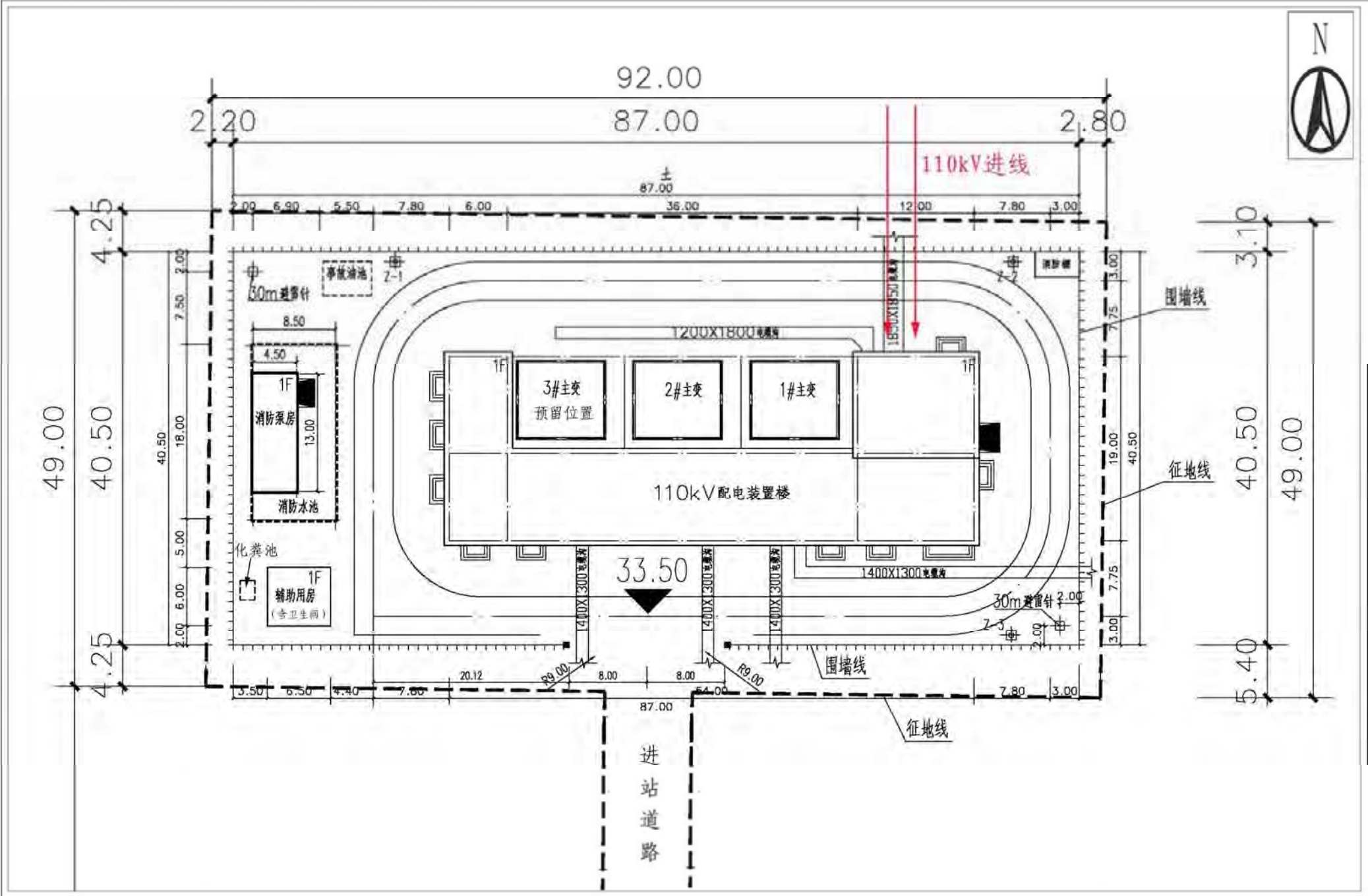
附图4 110kV翔西站总平面布置图 比例尺1: 500
