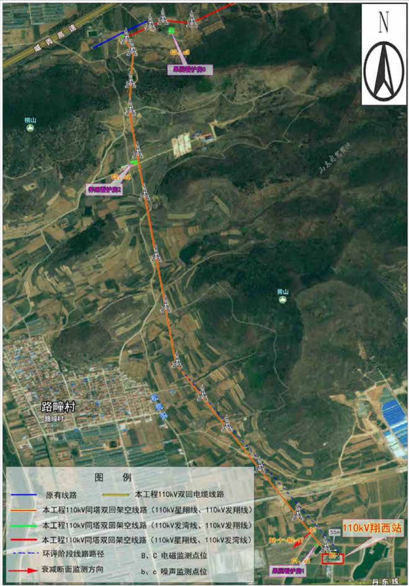
附图3(a) 本工程110kV输电线路路径及周边关系影像图 比例尺1:10000
