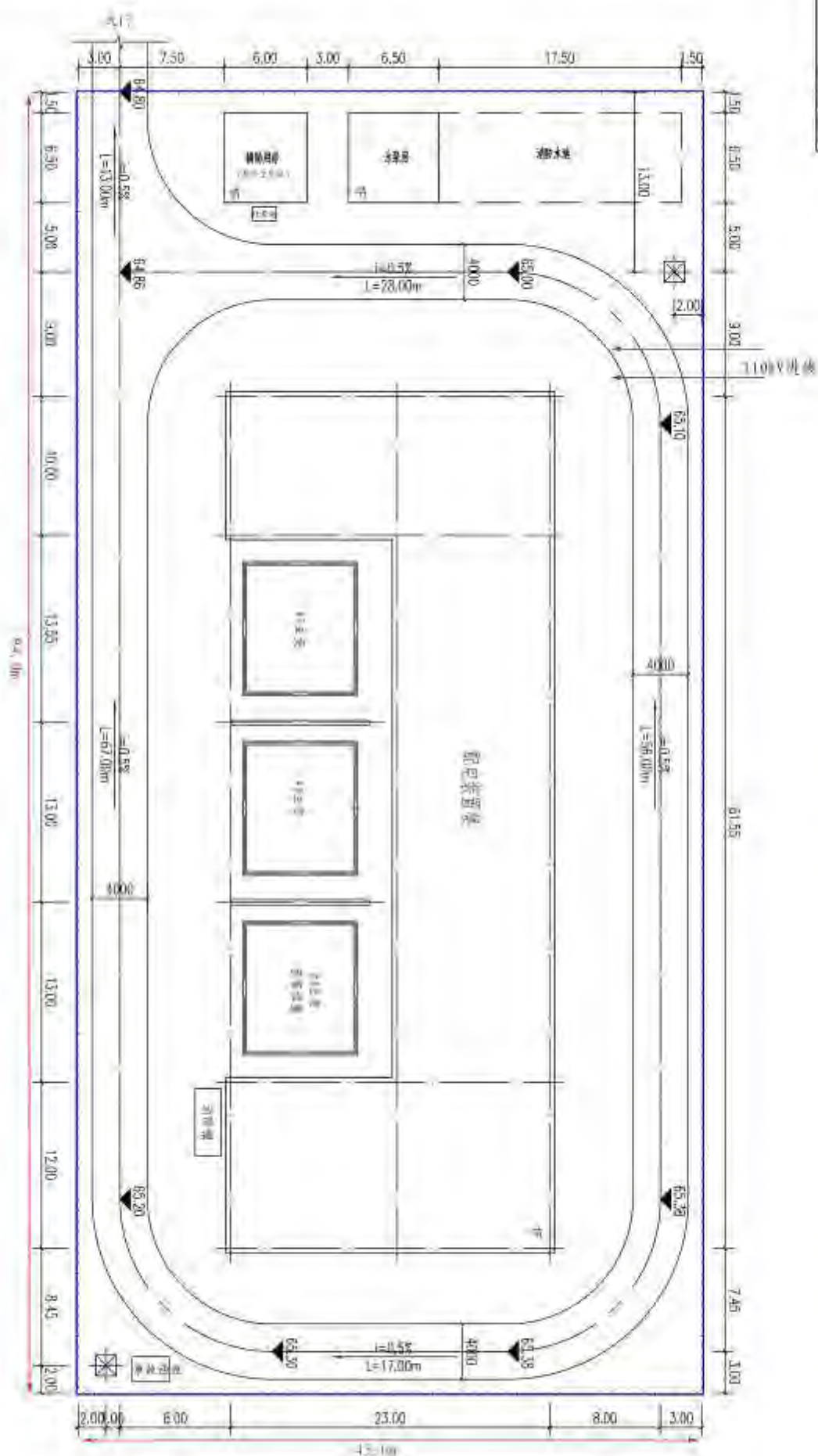
附图4 110kV蒋双站平面布置图 比例尺1:430
