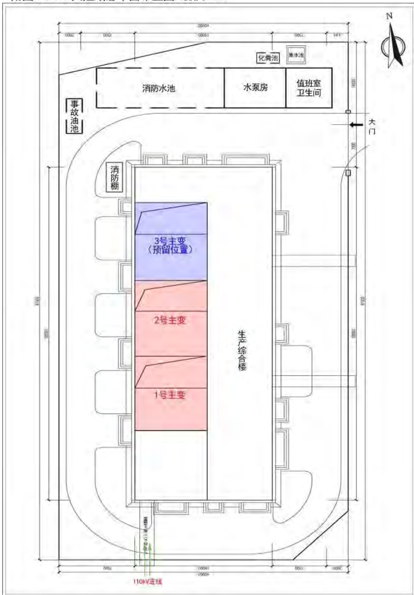
附图3 110kV兴隆站总平面布置图 比例尺1:330
