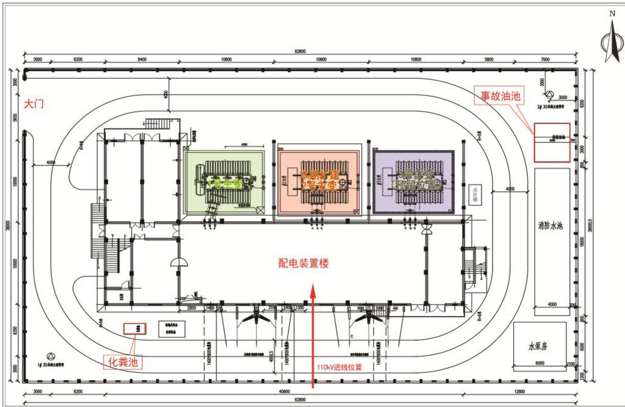
附图3 本工程变电站总平面布置图 比例尺1:300
